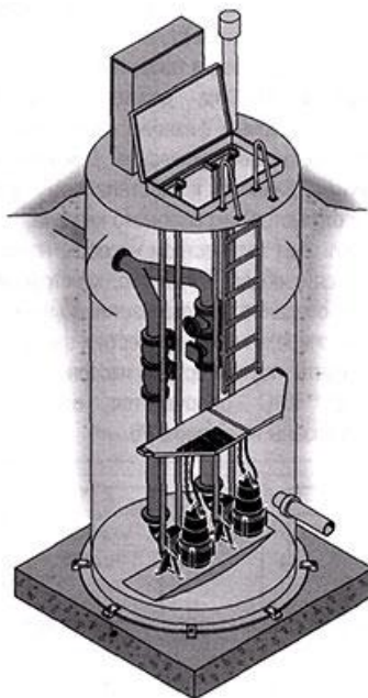
Рис.7. Комплектные канализационные насосные станции Grundfos
